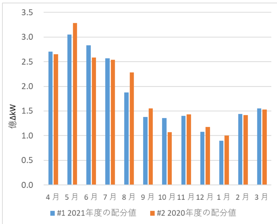
三次②必要量（月別）
