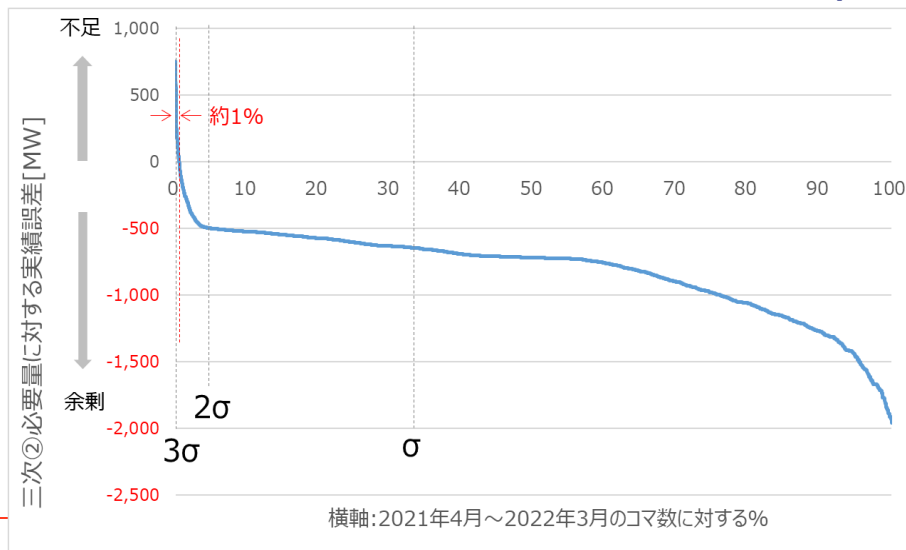
『三次②必要量+電源Ⅰ(予測誤差分)』に対する 『実需給における予測誤差(前日予測値-実績値)』のデユレーションカーブ (縦軸：前日予測値 - 実績値 - 三次②必要量 - 電源Ⅰ(予測誤差分))
