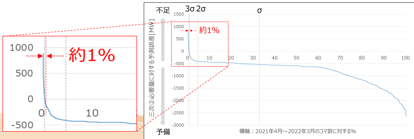
『三次②必要量+電源Ⅰ(予測誤差分)』に対する『実需給における予測誤差(前日予測値－実績値)』のデレーションカーブ (縦軸：前日予測値－実績値－三次②必要量－電源Ⅰ(予測誤差分))
