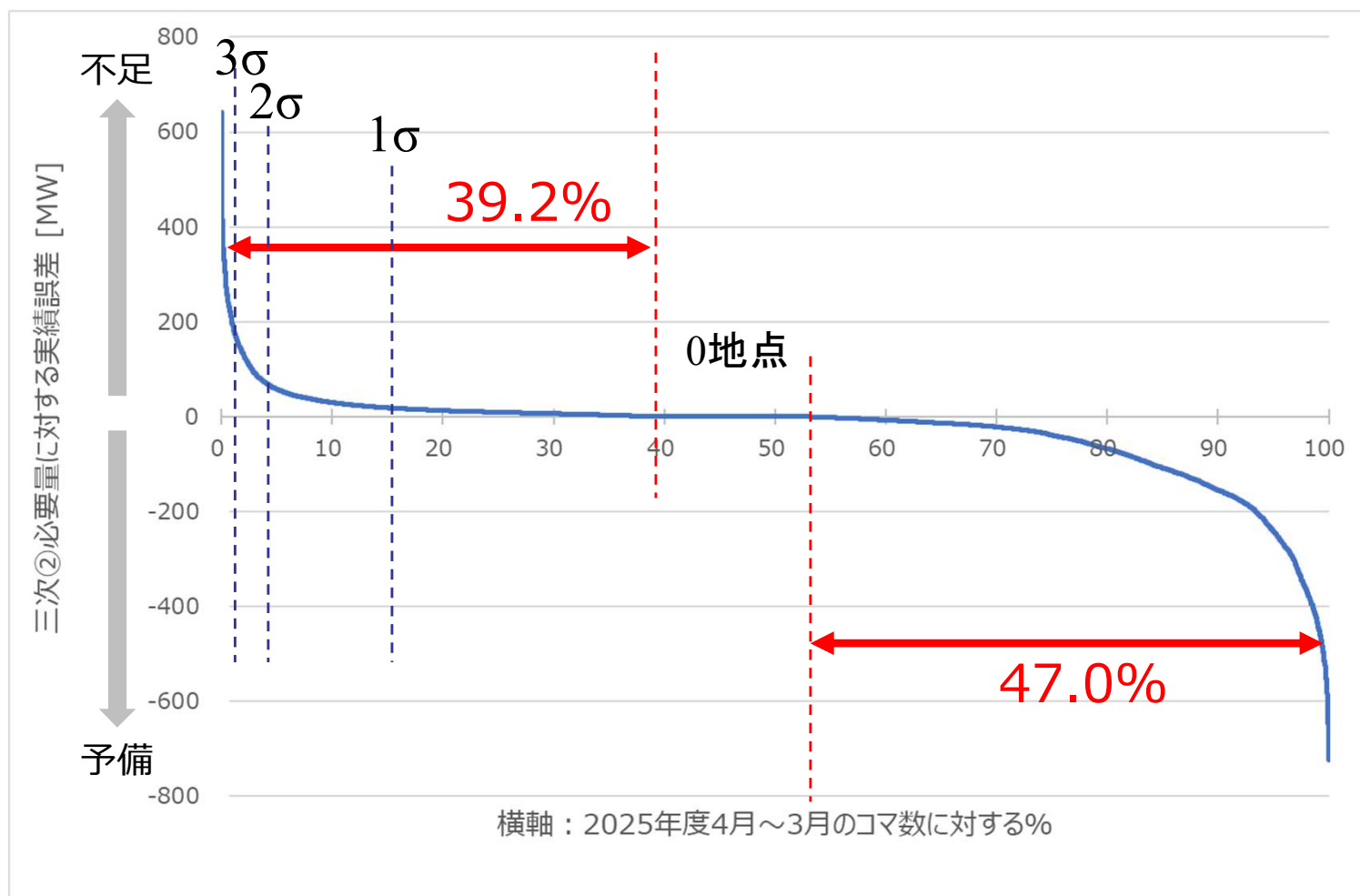
三次②必要量に対する予測誤差のデュレーションカーブ (縦軸：前日予測値－GC予測値－三次②必要量)
